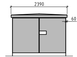
FASAD MOT D SKALA A1=1:50 A3=1:100
