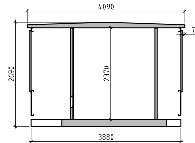
SEKTION A-A SKALA A1=1:50 A3=1:100
