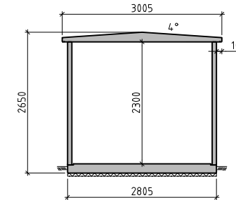
SEKTION A-A SKALA A1=150 A3=1:100
