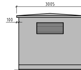
FASAD MOT D SKALA A1=150 A3=1:100
