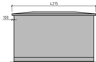
FASAD MOT A SKALA A1=150 A3=1:100
