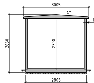
SEKTION A-A SKALA A1=1:50 A3=1:100
