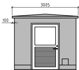
FASAD MOT B SKALA A1=1:50 A3=1:100
