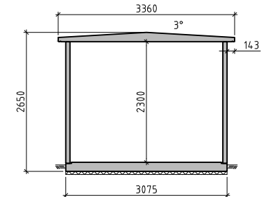
SEKTION A-A SKALA A1=1:50 A3=1:100
