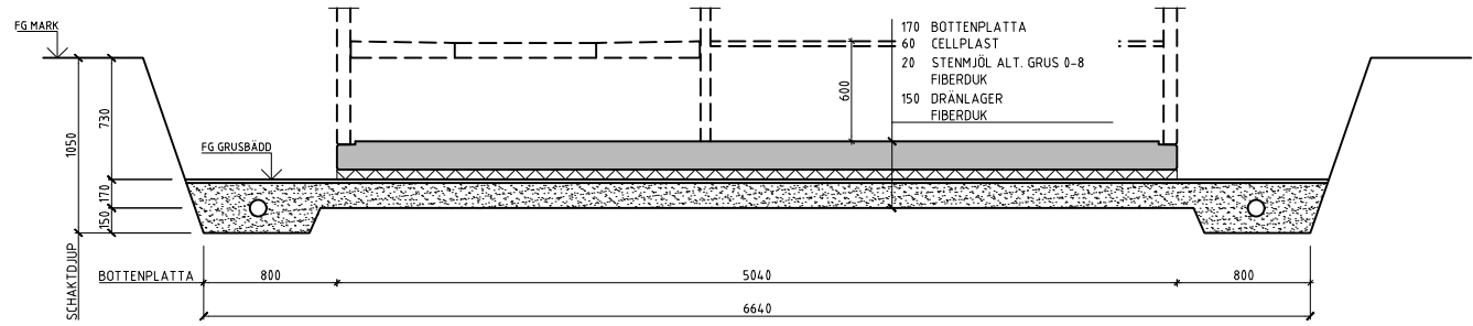
SEKTION A-A SKALA 1:20
