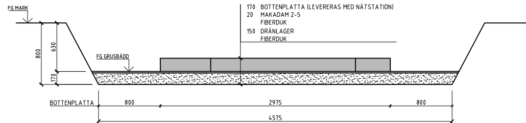
SEKTION A-A SKALA 1:20
