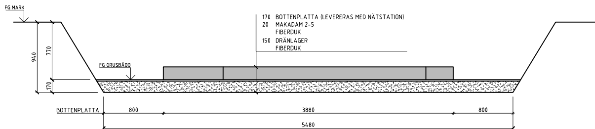
SEKTION A-A SKALA 1:20
