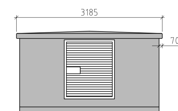
FASAD MOT A SKALA A1=150 A3=1:100
