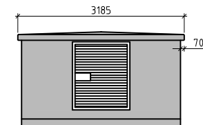
FASAD MOT A SKALA A1=1:50 A3=1:100
