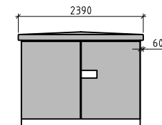
FASAD MOT B SKALA A1=1:50 A3=1:100
