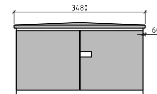
FASAD MOT D SKALA A1=1:50 A3=1:100
