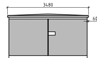
FASAD MOT B SKALA A1=1:50 A3=1:100
