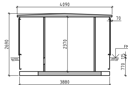
SEKTION A-A SKALA A1=1:50 A3=1:100
