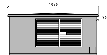
FASAD MOT A SKALA A1=1:50 A3=1:100
