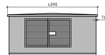
FASAD MOT C SKALA A1=1:50 A3=1:100
